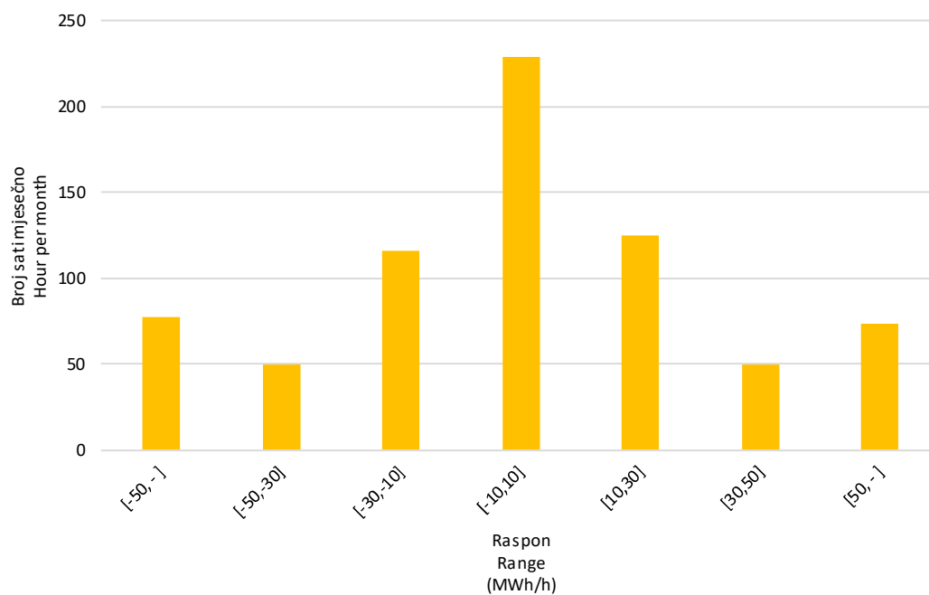
Slika 10 Statistička raspodjela satnih promjena proizvodnje VE u studenom 2025. godine
