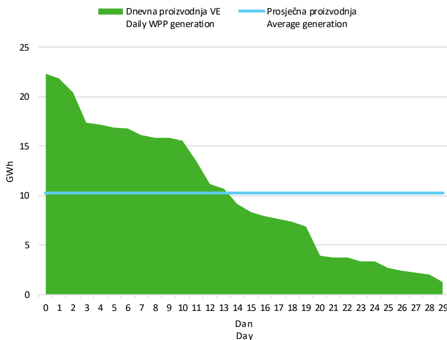
Slika 6 Krivulja trajanja dnevne proizvodnje vjetroelektrana u studenom 2025. godine
