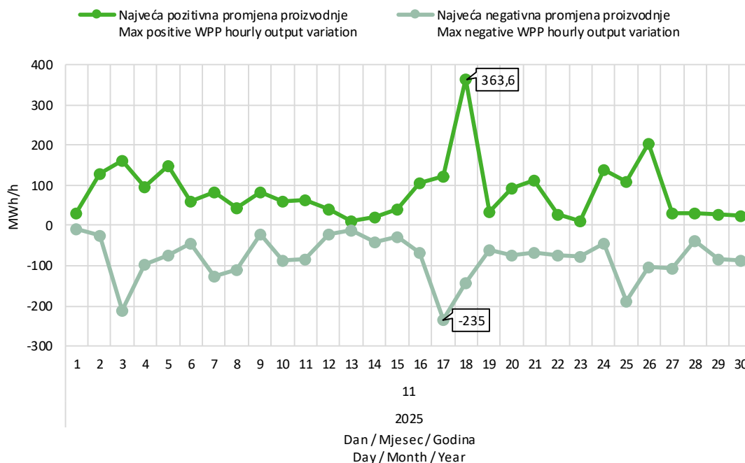
Slika 9 Maksimalna pozitivna i maksimalna negativna promjena satne proizvodnje VE u studenom 2025. godine
