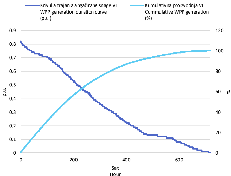
Slika 3 Krivulja trajanja angažirane snage svih VE i kumulativna proizvodnja VE u studenom 2025. godine u jediničnim vrijednostima
