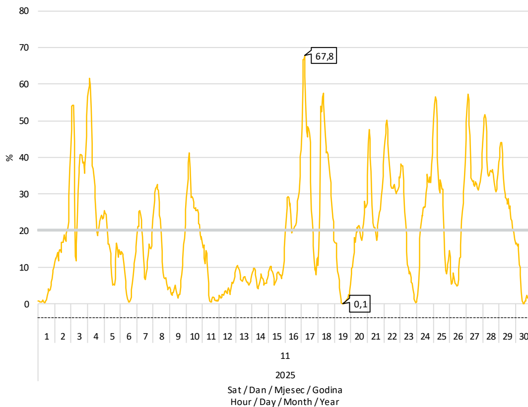
Slika 8 Udio proizvodnje vjetroelektrana u pokrivanju satnog opterećenja elektroenergetskog sustava u studenom 2025. godine
