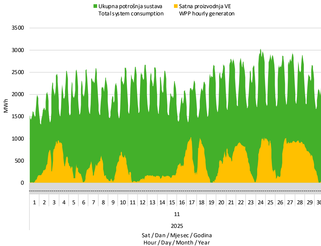
Slika 7 Usporedba satnog dijagrama opterećenja sustava i proizvodnje vjetroelektrana u studenom 2025. godine
