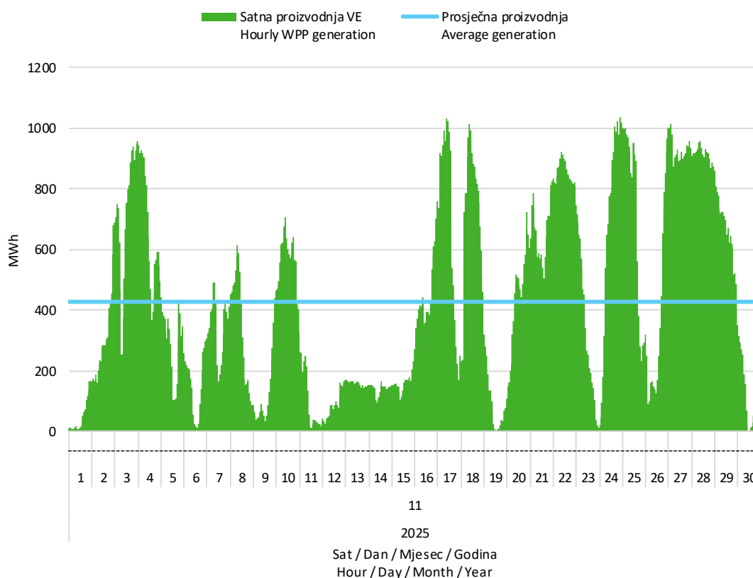
Slika 2 Satna proizvodnja svih vjetroelektrana u studenom 2025. godine
